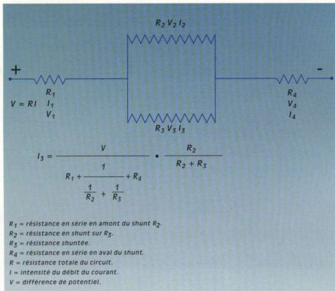
Figure 17 A. Effet de vol et circuit électrique. Le débit du courant dans chaque résistance en parallèle est proportionnel à la différence de potentiel entre les deux bornes du générateur moins la différence de potentiel entre les extrémités de la résistance d'amont en série, ainsi qu'au rapport entre les autres résistances en série et elle-même. Cela veut dire que la perte d'intensité dans chacune des résistances en série reste proportionnellement la même, quel que soit le rapport aux autres résistances en série et qu'il n'y a pas de vol de l'une par l'autre, mais que c'est la résistance d'amont en série qui « vole » plus ou moins du courant selon son importance en faisant chuter la tension. On ne peut faire varier l'intensité (le débit de courant) en R_2 et R_3 qu'en changeant les valeurs de R_1 . On voit aussi, selon la formule conforme à la loi d'Ohm, que si l'on considère que R_2 est le shunt, le débit ou intensité I_3 variera dans la direction R_2 dans les
